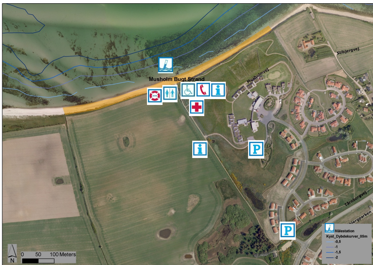
Figur 1. Musholm Bugt Strand med dybdekurver (0,5 til 2,0 meter).
