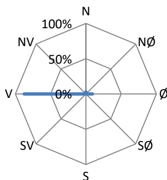
Figur 1. Strømretning (fra, %), Musholm Bugt Strand
