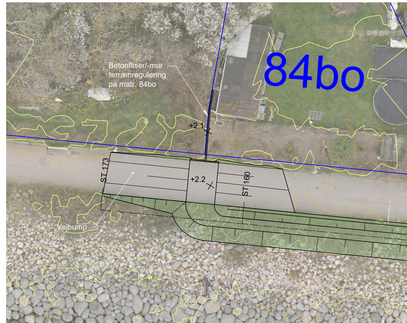
PLAN, 1:200 Vejbump. Bredde 3,8m. Anlæg 1:20
