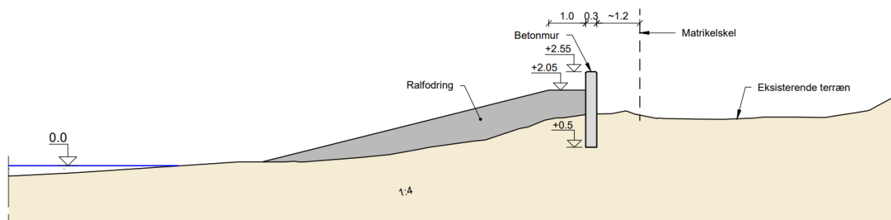
SNIT D-D, 1:100
