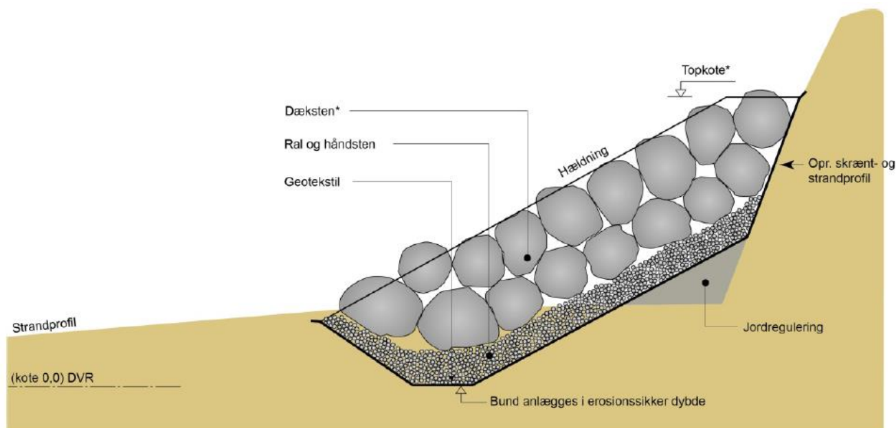
Figur 2.3: Principkitse fra kystdirektoratets beskrivelse af skråningsbeskyttelse
