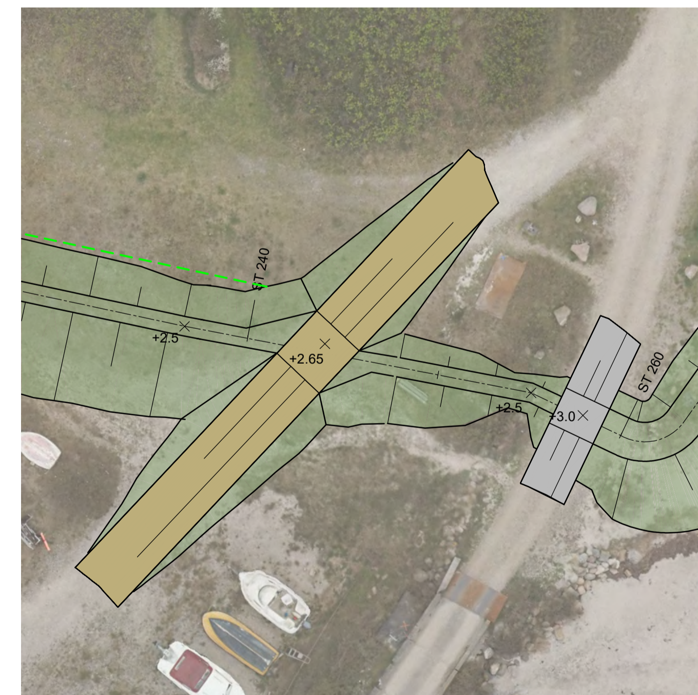
PLAN, 1:200 Overkørsel over dige. Bredde 3,0m. Anlæg 1:10 Vejbump på mole. Bredde 3,0m. Anlæg 1:5
