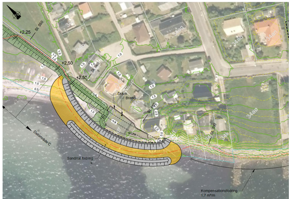
Figur 4-18 Plantegning af kystbeskyttelsen i område C. Det fremgår at kystbeskyttelsen optager areal fra matrikel 84df og 84dg. Se Tegn. Nr. C3_403.
