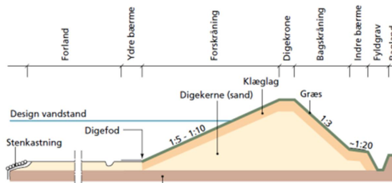
Figur 4-5 Principsnit i dige med flad forskrånning. Kilde: Kystdirektoratet.
