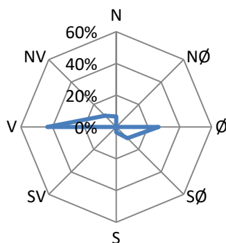
Figur 1. Strømretning (fra, %), Revkrogen Strand.
