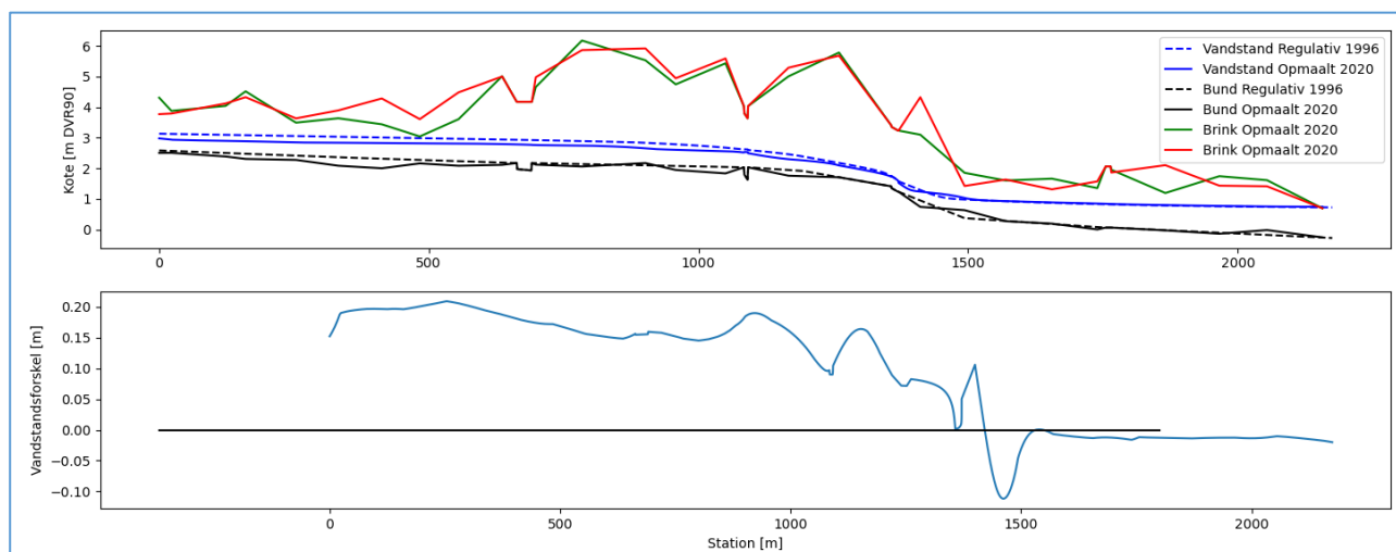
Fig 4: Øverst er vist sammenligning mellem beregnede vandstande for opmålt geometri og regulativmæssig geometri. Afstrømning på 32 \text{ l/s/km}^2 (vinter maksimum median) og Manningtal 25. Nederst er vist forskellen mellem de to vandstandskurver i øverste plot.
